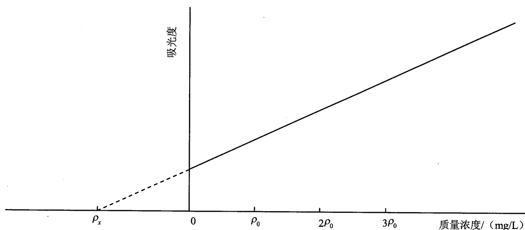
附图 B.1 待测试样质量浓度与对应吸光度的关系图
